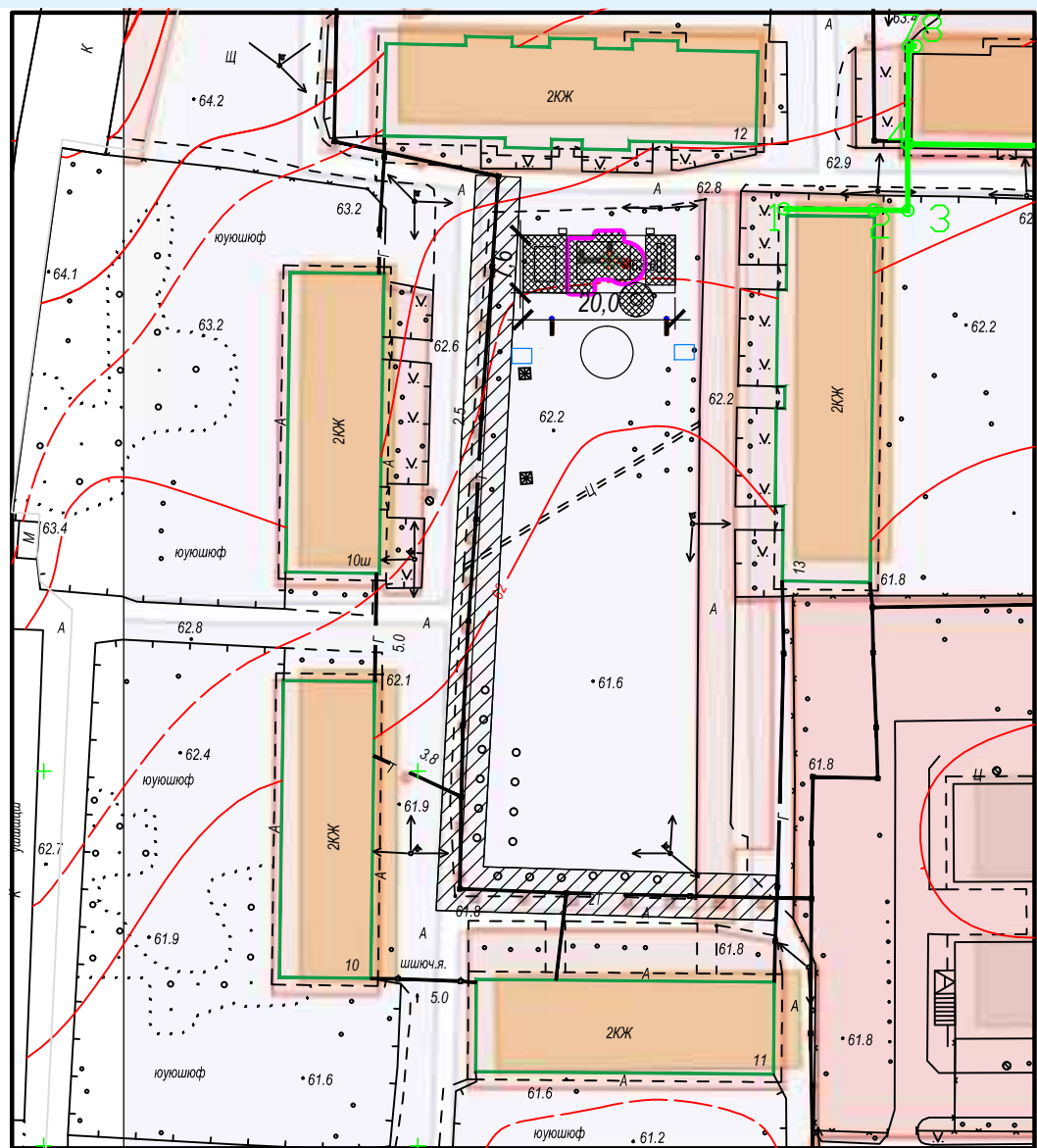
ГЕНЕРАЛЬНЫЙ ПЛАН БЛАГОУСТРОЙСТВА М1:1000
